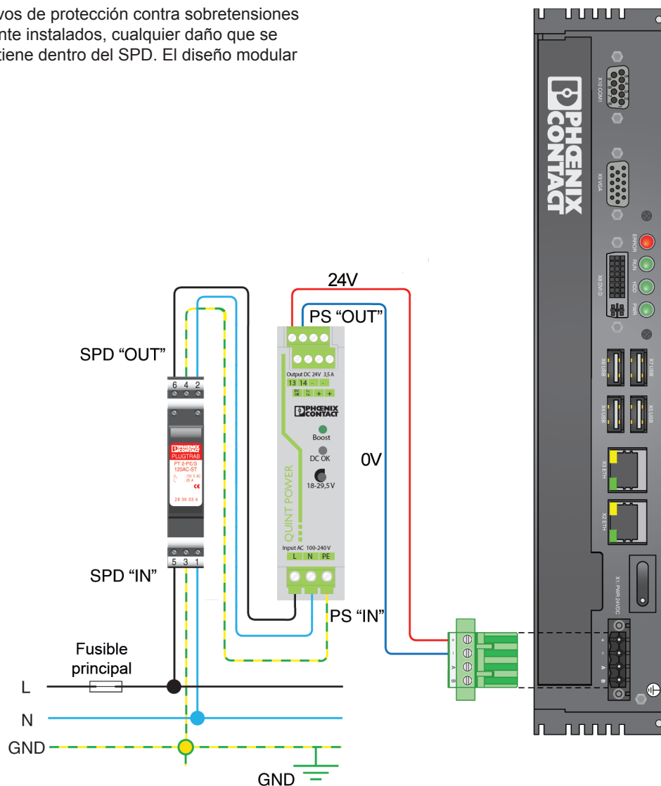
Imagen 1. Instalación típica de PC industrial Valueline
